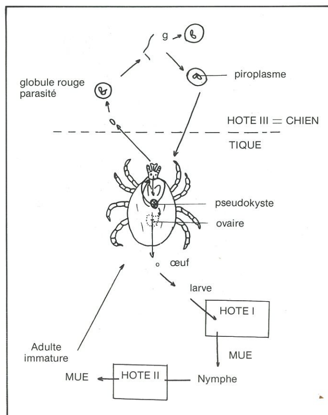
Fig. 1 — SCHÉMA DU CYCLE ÉVOLUTIF DE BABESIA CANIS ET DU CYCLE ÉVOLUTIF DES TIQUES
