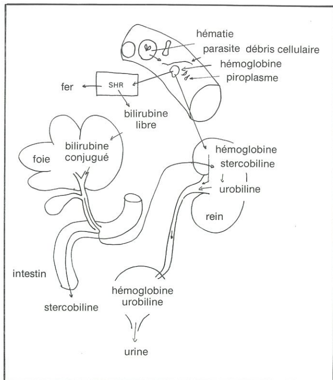
Fig. 2 — SCHÉMA PATHOGÉNIQUE DE LA PIROPLASMOSE
